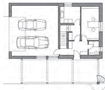
Půdorys přízemí
