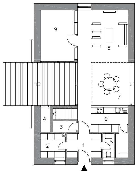
Půdorys přízemí
