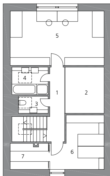
Půdorys poschodí
