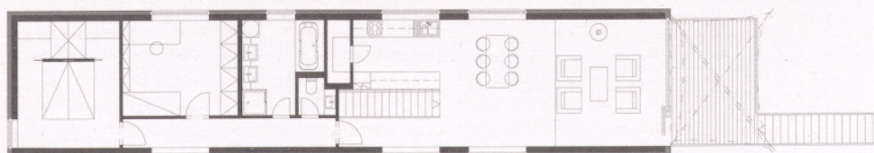
půdorys 1. NP
