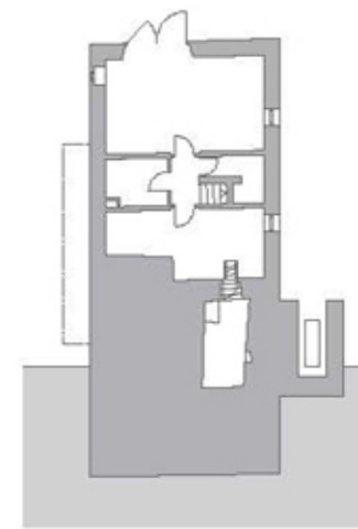
Pôdorys 1. pp
